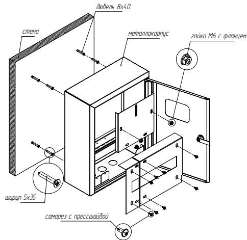
Рис. 1 - Схема монтажа
